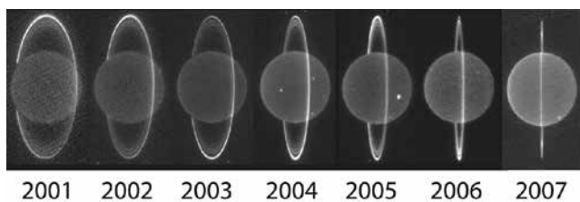
De Planeet Uranus, in verschillende jaren gefotografeerd. Duidelijk is te zien dat de Planeet 'op zijn zij' ligt.
