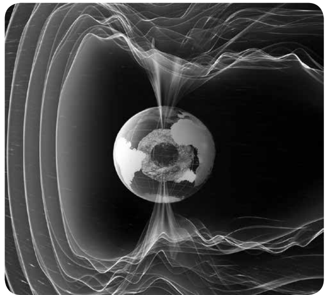
Een voorstelling van het magnetische veld van de Aarde; de Zonnewind (in deze tekening van links komend) vervormt het veld sterk.
